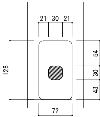
受け側
